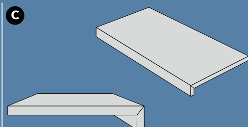
C ELEMENTO PROFILO A "L" INCOLLATO BONDED "L" PROFILE ELEMENT PROFILÉ EN « L » COLLÉ GEKLEBTES „L“-PROFILELEMENT
